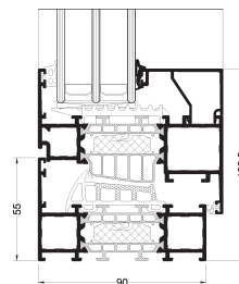
GT ablak keresztmetszet
