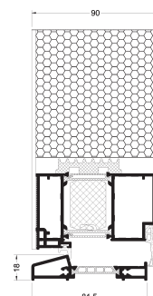
Panelajtó keresztmetszet kétoldalas panel, befelé nyíló
