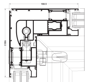
UG 90°-os sarokmegoldás keresztmetszet
