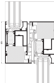
UG i+ keresztmetszet
