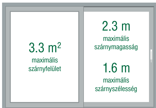
Toló-bukó erkélyajtók méréthatárai
